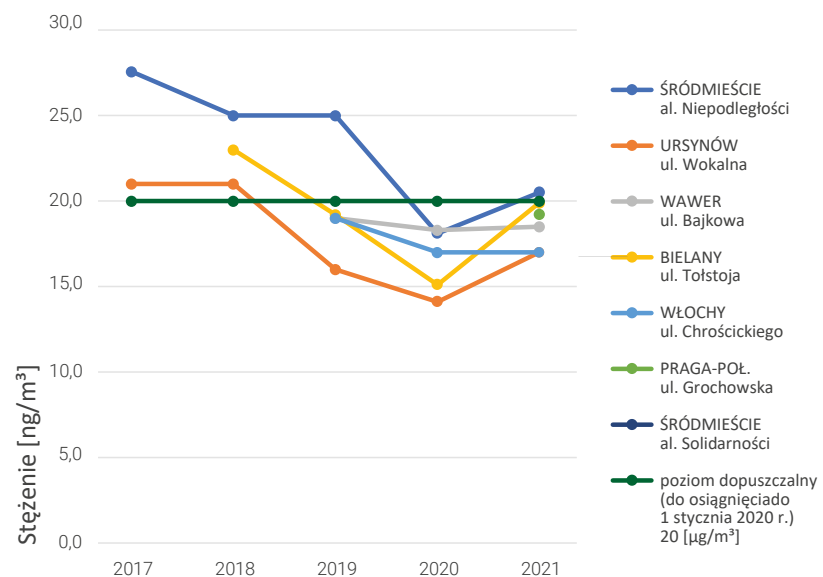
Stężenia średnioroczne pyłów zawieszonych PM 2,5 na stacjach pomiarowych w Warszawie 2017-2021
