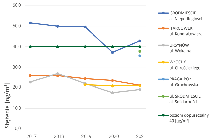
Stężenia średnioroczne dwutlenku azotu NO 2 na stacjach pomiarowych w Warszawie
