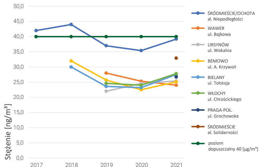
Stężenia średnioroczne pyłów zawieszonych PM10 na stacjach pomiarowych w Warszawie 2017-2021
