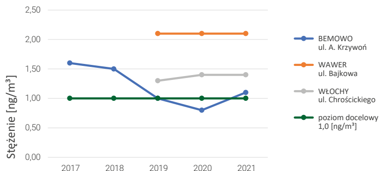
Stężenia średnioroczne benzo(a)pirenu na stacjach pomiarowych w Warszawie
