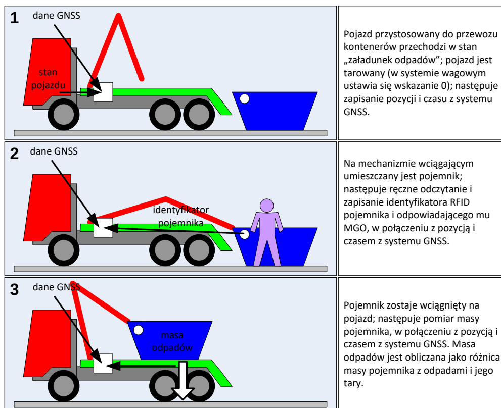
rys. 6 „załadunek odpadów połączone z ważeniem” – pojazd hakowy
