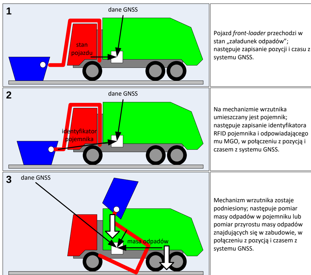
rys. 9 „załadunek odpadów połączone z ważeniem” – pojazd „front loader”
