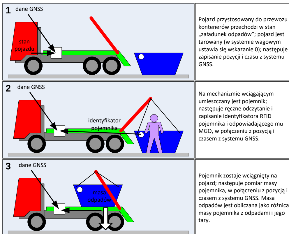
rys. 10 „załadunek odpadów połączone z ważeniem” – pojazd bramowy
